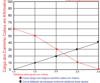
Gráfico Carga TS EN 61537(safety factor 1.7)
