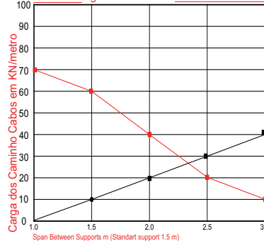
Gráfico Carga TS EN 61537(safety factor 1.7)
